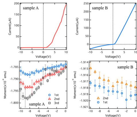
図 3. Pd/酸素ドーパド STO の I - V 曲線と磁化の電圧依存性。
