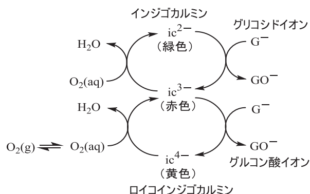
図3. 信号反応系の概要。 \text{O}_2(\text{g}) は空気中の酸素, \text{O}_2(\text{aq}) は溶液中に溶けている酸素を意味する。
