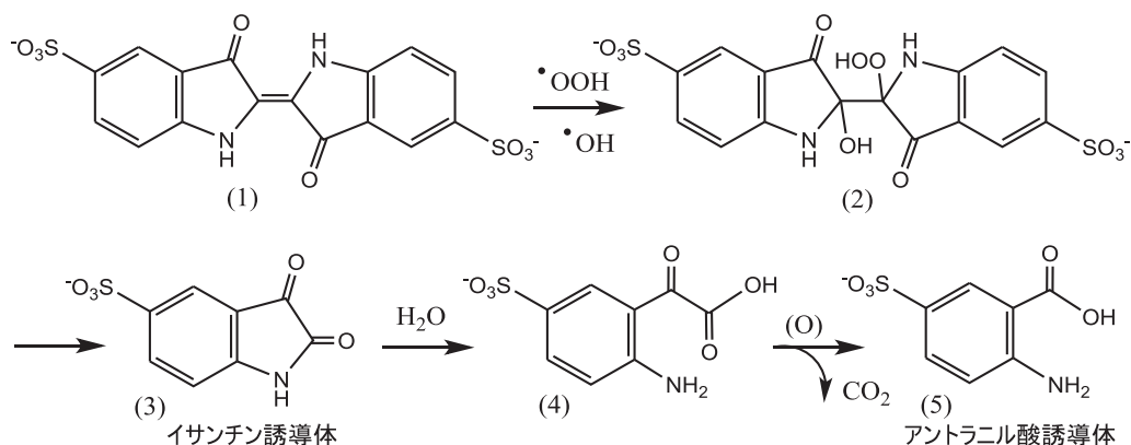
図10. インジゴカルミンの過酸化水素による分解反応
