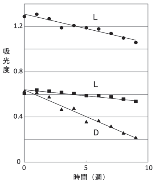
図 12. インジゴカルミン水溶液の退色。吸収帯 ( \lambda_{\max} = 610 \text{ nm} ) における吸光度の時間変化を、2 種類の濃度について示している。L は日常の室内照明下、D は遮光して保存（室温 22 ～ 27 °C）。
