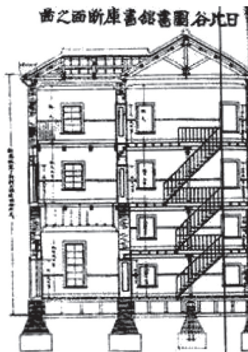
第6図 断面図 2)
