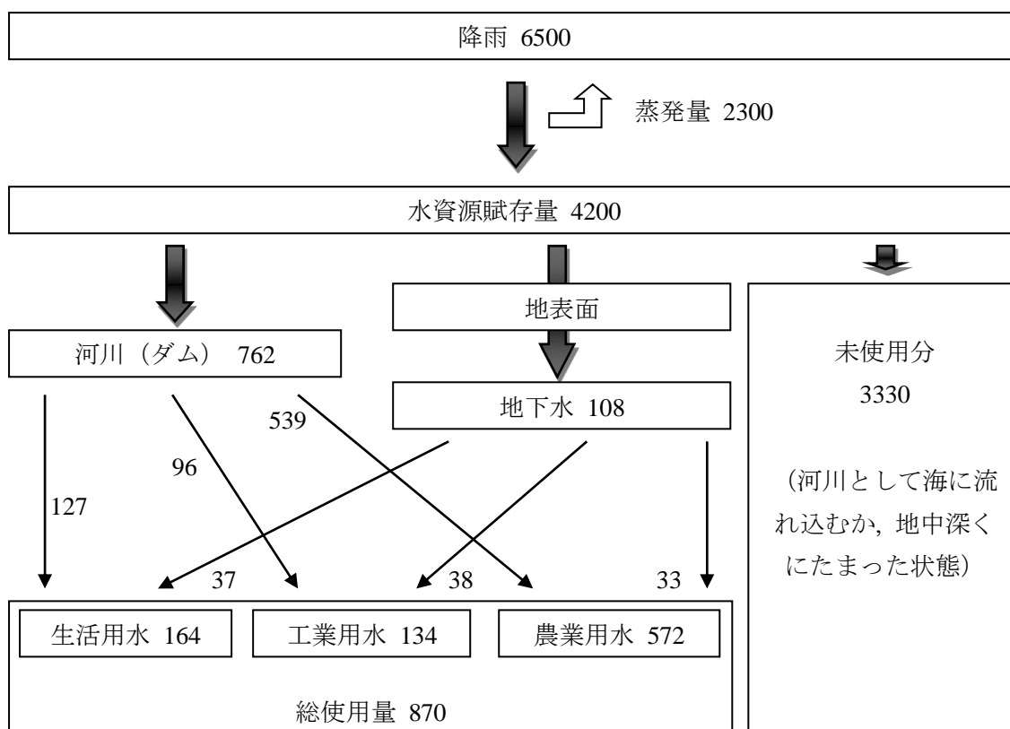
図 10 日本の水収支（平成 12 年）
