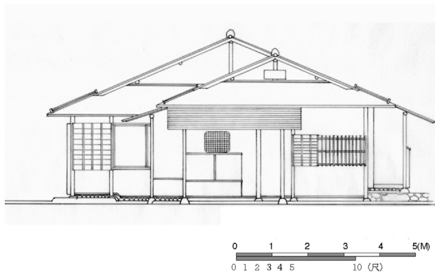
図4 S邸立面図
