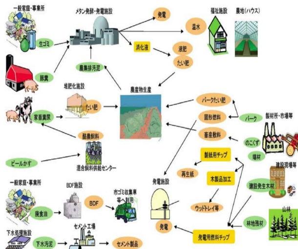
日田市バイオマスタウン構想におけるバイオマス利活用フロー図 日田市HP
