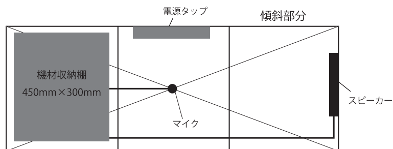
図 4.26: 機材設置図
