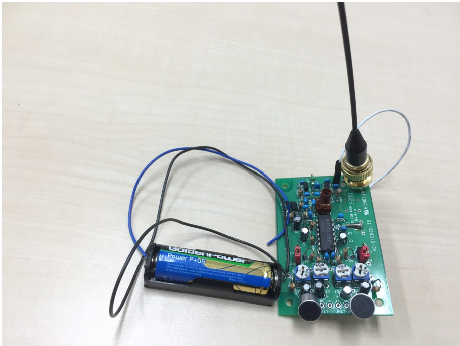
図 3.18: 送信機
