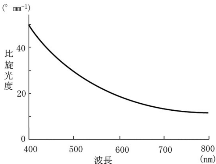
図2. 右旋性石英の比旋光度の波長依存性
