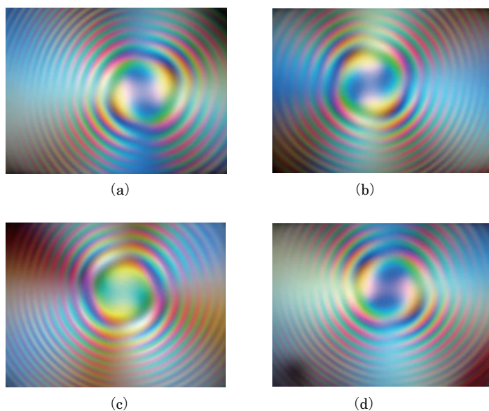
図18. 水晶板のコノスコープ像（偏光子の透過軸は水平方向で，検光子として円偏光板を使用）。(a) 左水晶（左円偏光），(b) 左水晶（右円偏光），(c) 右水晶（左円偏光），(d) 右水晶（右円偏光）。
