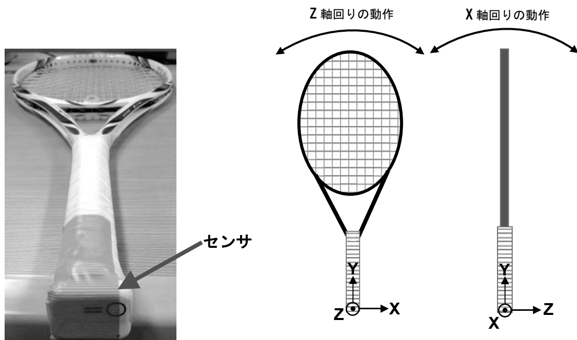
図2 センサの取り付け位置と、X軸、Z軸の定義
