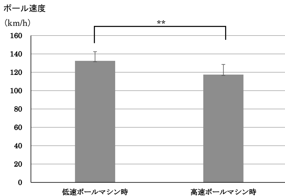
図 5 低速ボールマシンから出たボールを打ったときと、高速ボールマシンから出たボールを打ったときのボール速度 (平均値 + 標準偏差) ** < 0.01
