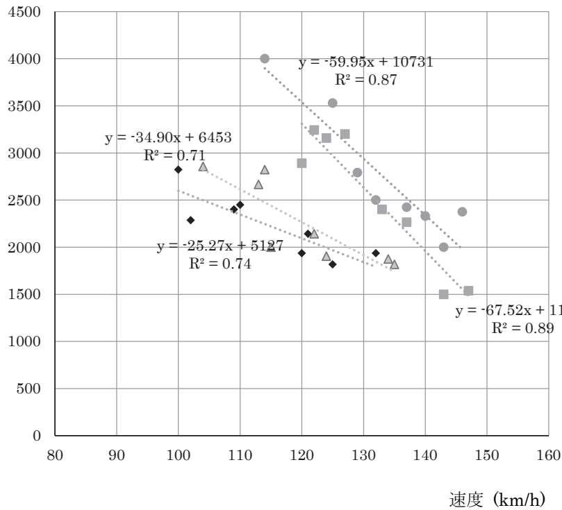
図11 「右奥」を狙ったときと「左奥」を狙ったときのボール速度 - 回転量関係の比較
