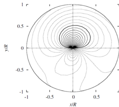
図4 旋回培養器中の細胞の半径方向速度コンター [雑誌論文①, 図書①]
