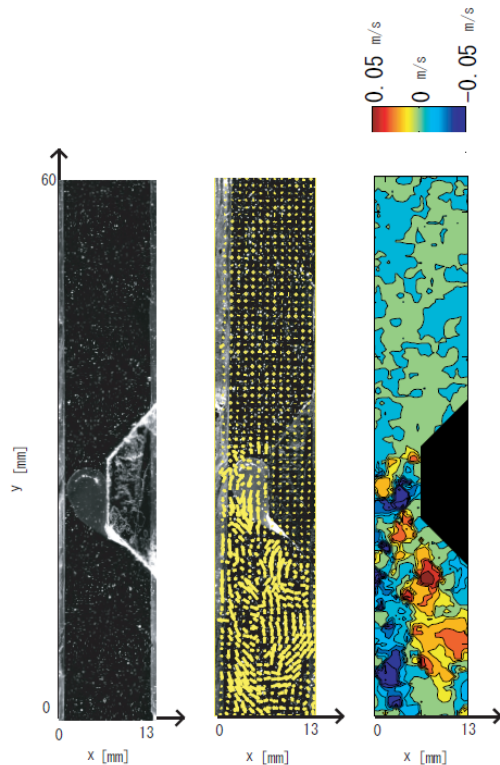
図 7 縮小・流路中のグリセリン液滴の挙動：(左) カメラによる取得画像 (中) PIV 処理によって得られた速度ベクトル場 (右) 同・速度場コンター [学会発表②]
