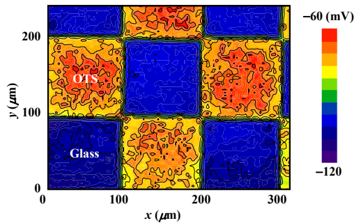
図2 壁面ゼータ電位パターンの一例。
