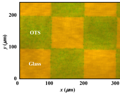
図1 電位時空間分布カラーイメージングの一例。
