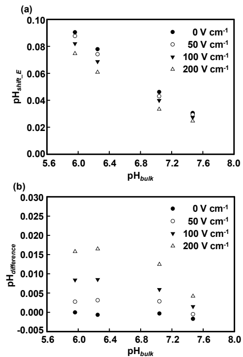
図4 バルクと壁面近傍のpH分布。
