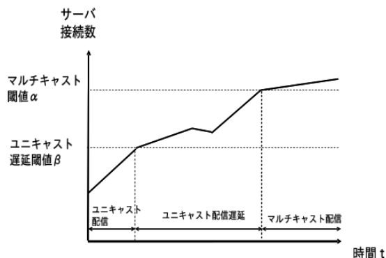
基本的には、従来通りユニキャスト配信を行い、単位時間内の同時接続数が閾値を超えた場合、ダウンロード開始のタイミングを調整（遅延）させるスケジュールドユニキャストに切り替える。新規接続を遅延させ、単位時間当たりの接続数を維持することにより、すでにダウンロード中のユーザのダウンロード速度を維持することが可能となる。スケジュールドユニキャスト中に、さらにサーバ接続要求が減少した場合は再度ユニキャストに戻すが、増大した場合はマルチキャスト
