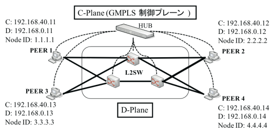
図 8 実装ネットワーク構成
