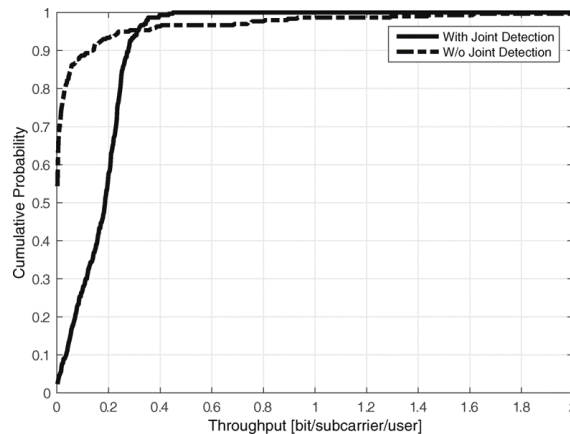
(b) ピコセルにおけるスループット特性
