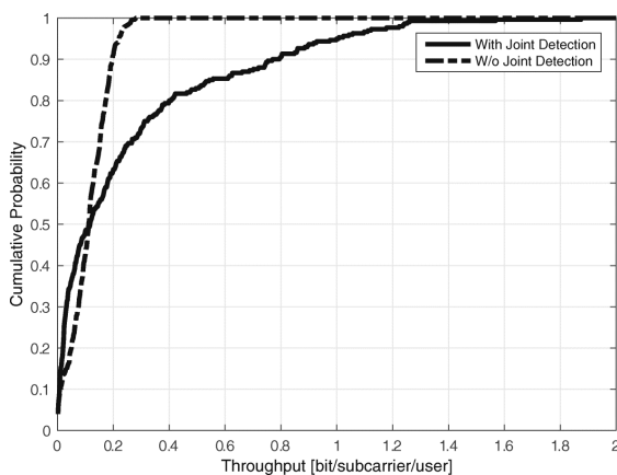
(a) マクロセルにおけるスループット特性
